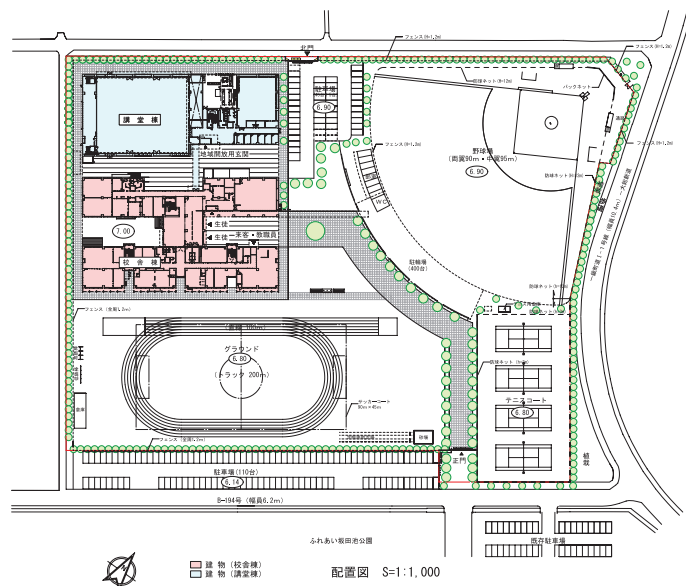
校舎とグラウンドの配置図
