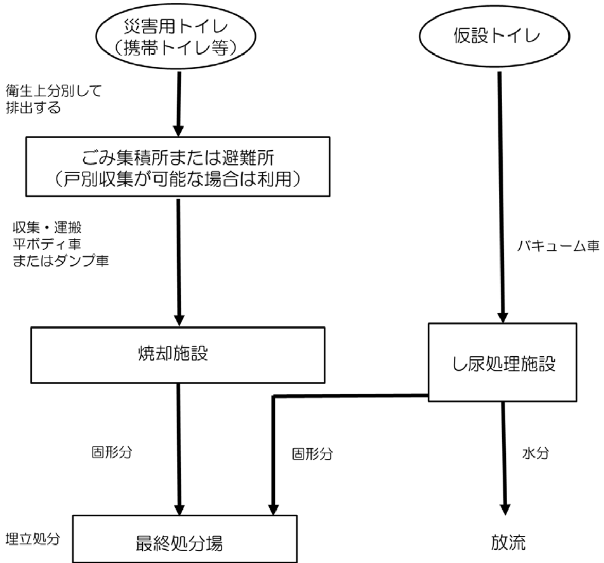
図表1-13 し尿処理の流れ
