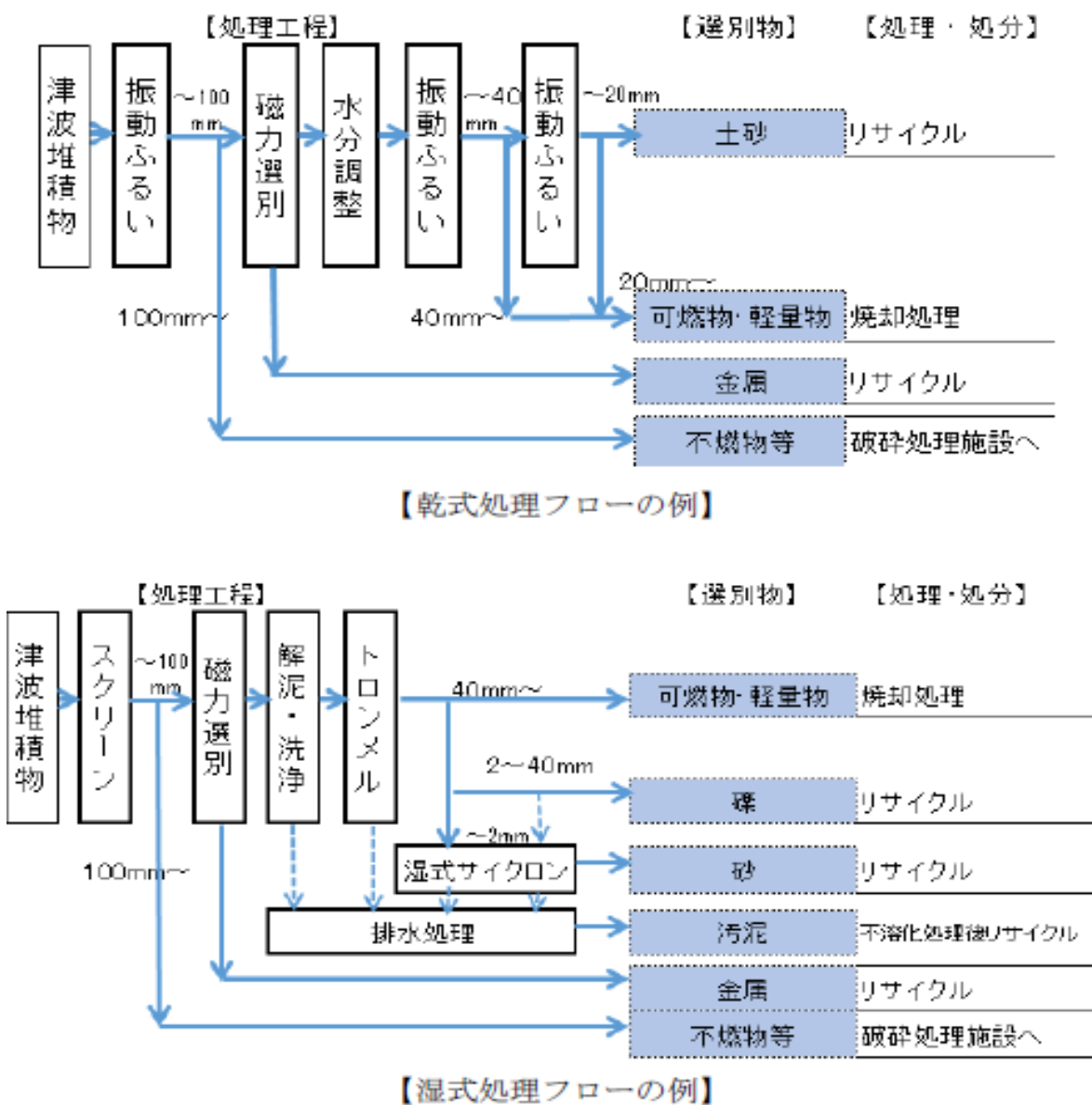
図表6-12 津波堆積物の処理（例）
