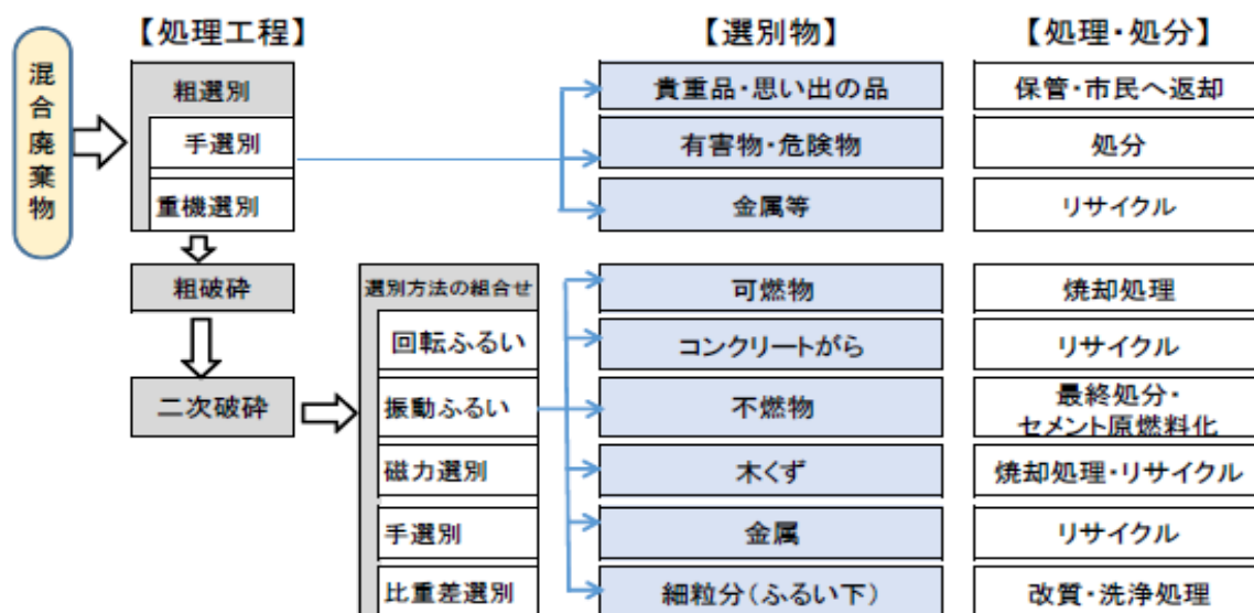
図表6-11 混合廃棄物の処理（例）
