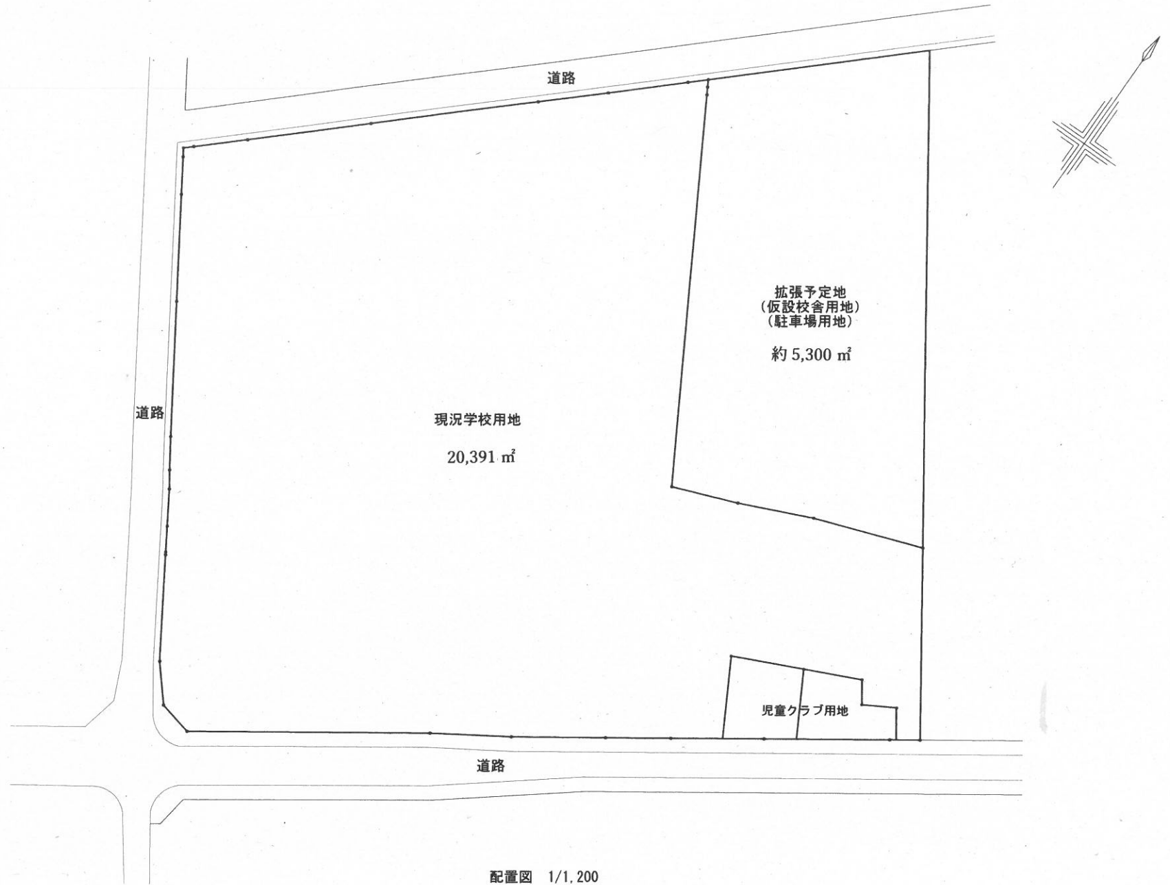
配置図 1/1,200
