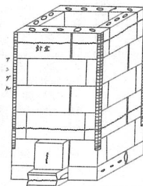
小型焼却炉
