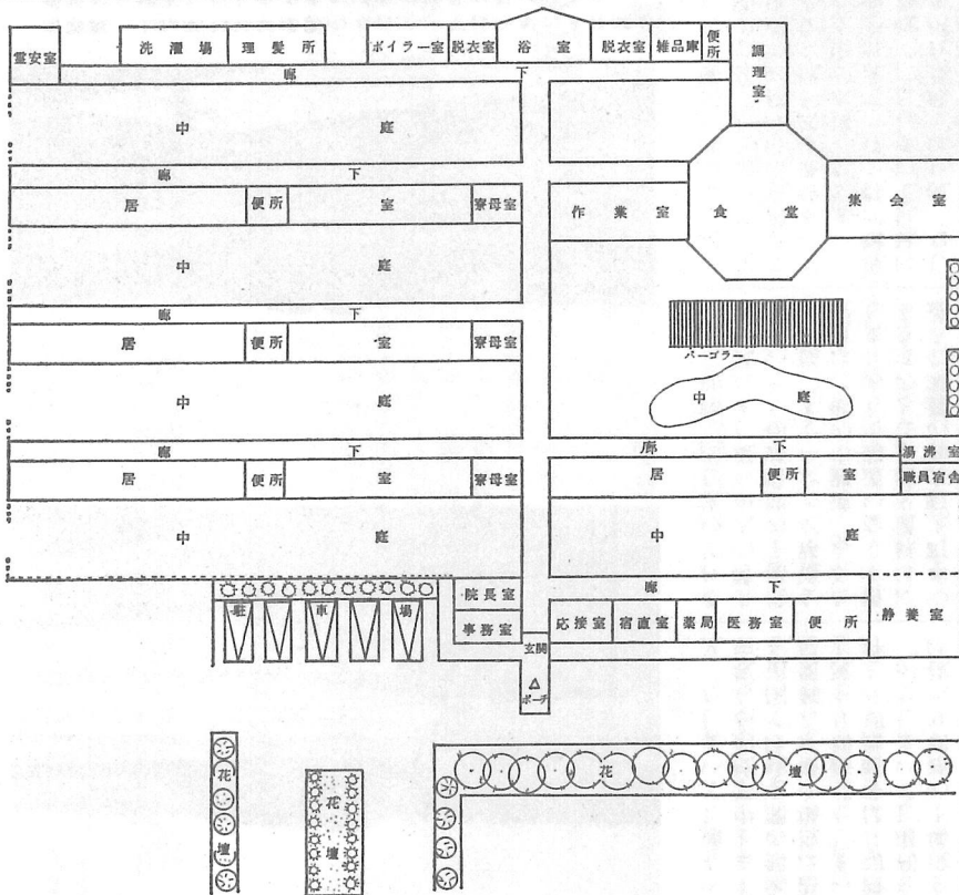
養護老人ホーム配置図
