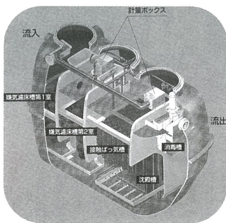
し尿と生活排水を処理する合併処理浄化槽
